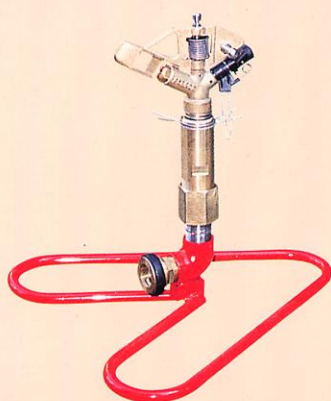
Zスプリンクラー付中型ベースセット MB-ZK30型 (ノズル3個付)
