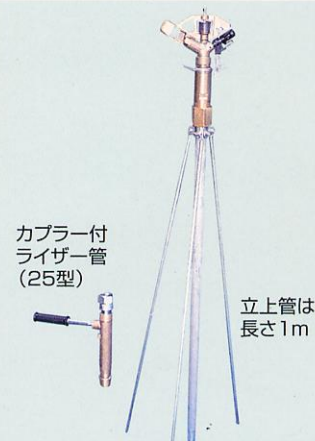
立上り管付スプリンクラー 3FR-ZK30型 (三脚付)
