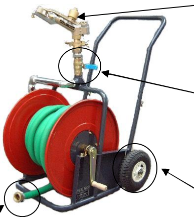
NSG30-2WL(グリーンホース仕様) ※グリーンホースは別売。口径・長さを指定してください。
